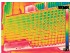
外壁タイル面浮き
